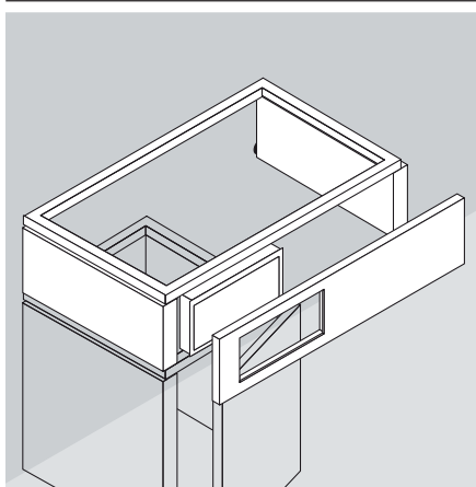
Abwurfklappe für den Einbau von hinten in Konsolblenden
